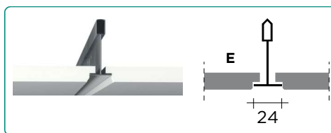
muchie E24 - structura retrasa
