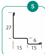
sectiune W 27 x 15 x 6 x 15 mm
