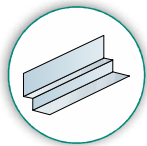
profil perimetral sectiune W 27 x 15 x 6 x 15 mm
