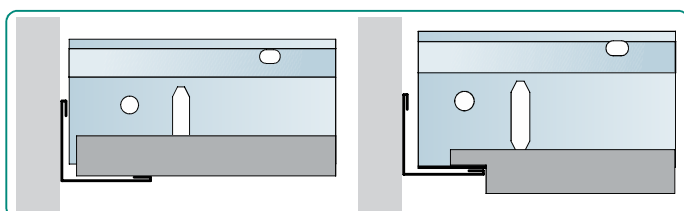
profil perimetral sectiune L 19 x 24 mm
