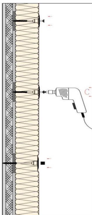
Instalare la suprafață cu dop STR
