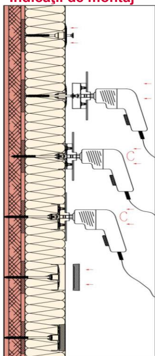
Montaj ascuns cont. principiului STR, cu rondea STR
