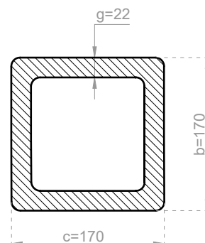
SECTIUNE TRANSVERSALA
