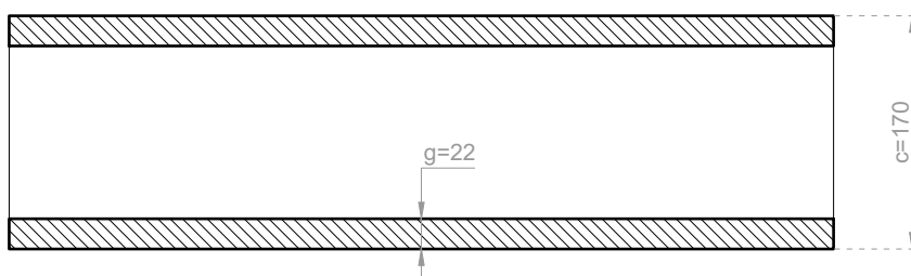
SECTIUNE LONGITUDINALA
