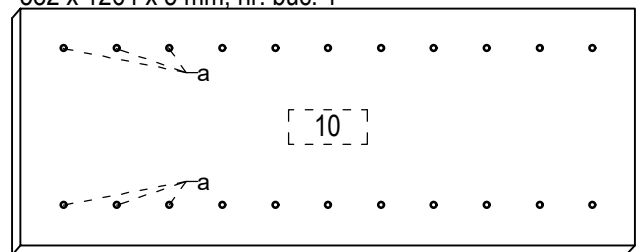
582 x 1264 x 5 mm; nr. buc: 1
