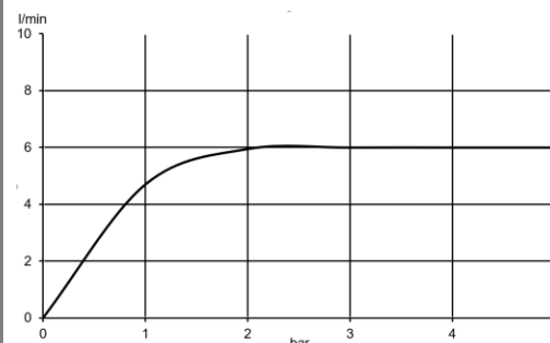
Diagramă debit
