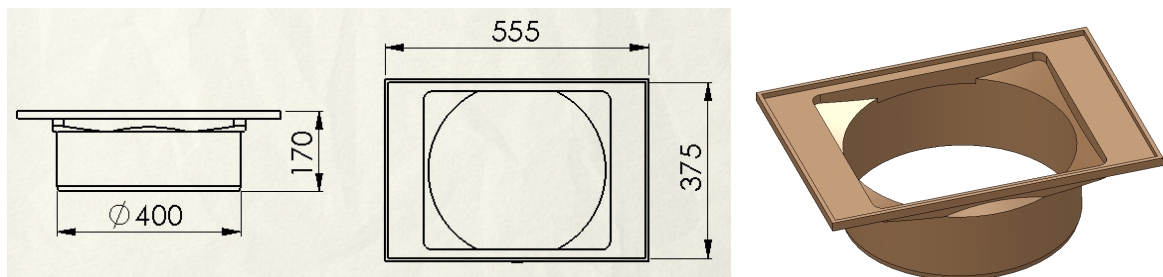
Fig. 2 Piesa de sprijin pentru gratar fonta clasa C250
