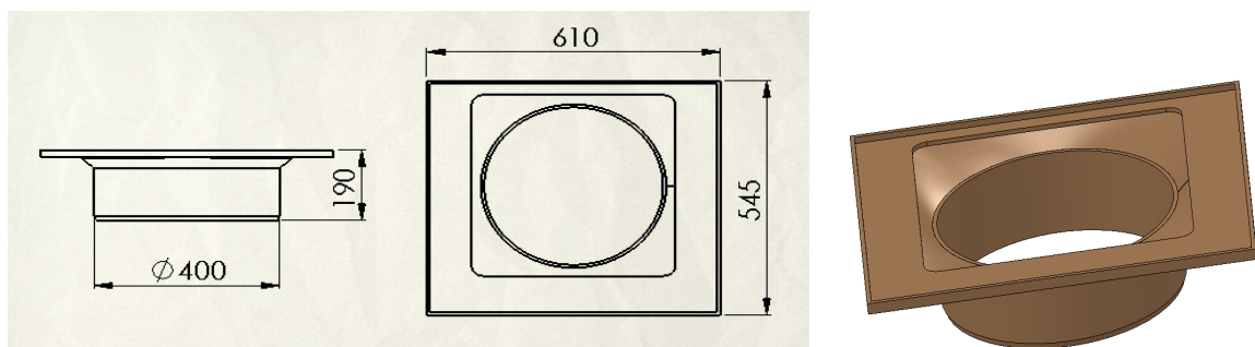
Fig. 3 Piesa sprijin pentru gratar fonta clasa D400
